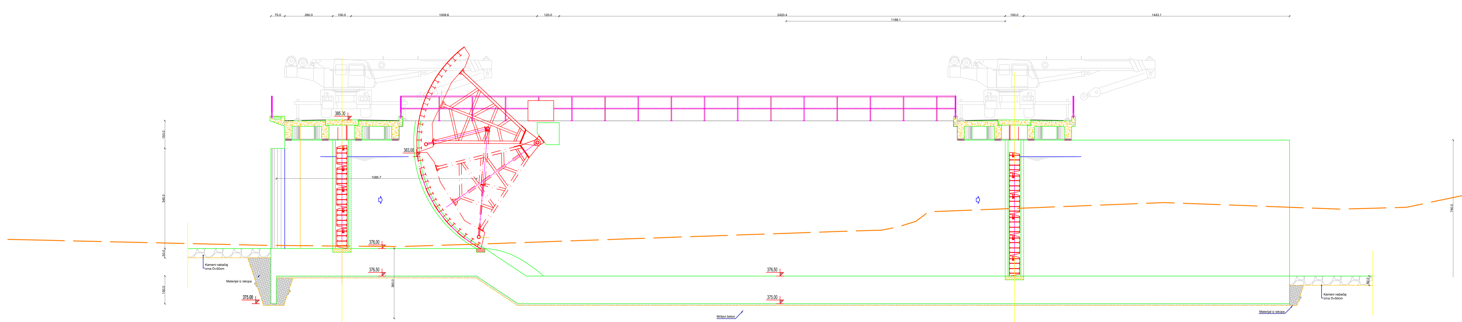
mHE Piskanja - Presek p5-p5
